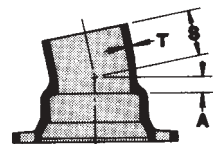
MJ & PE 11 1/4° Bend
