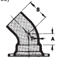
MJ x PE 45° Bend
