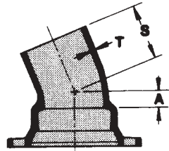
MJ x PE 22 1/2° Bend
