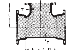
MJ x MJ x FLG Tee
