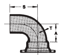
MJ x PE 90° Bend
